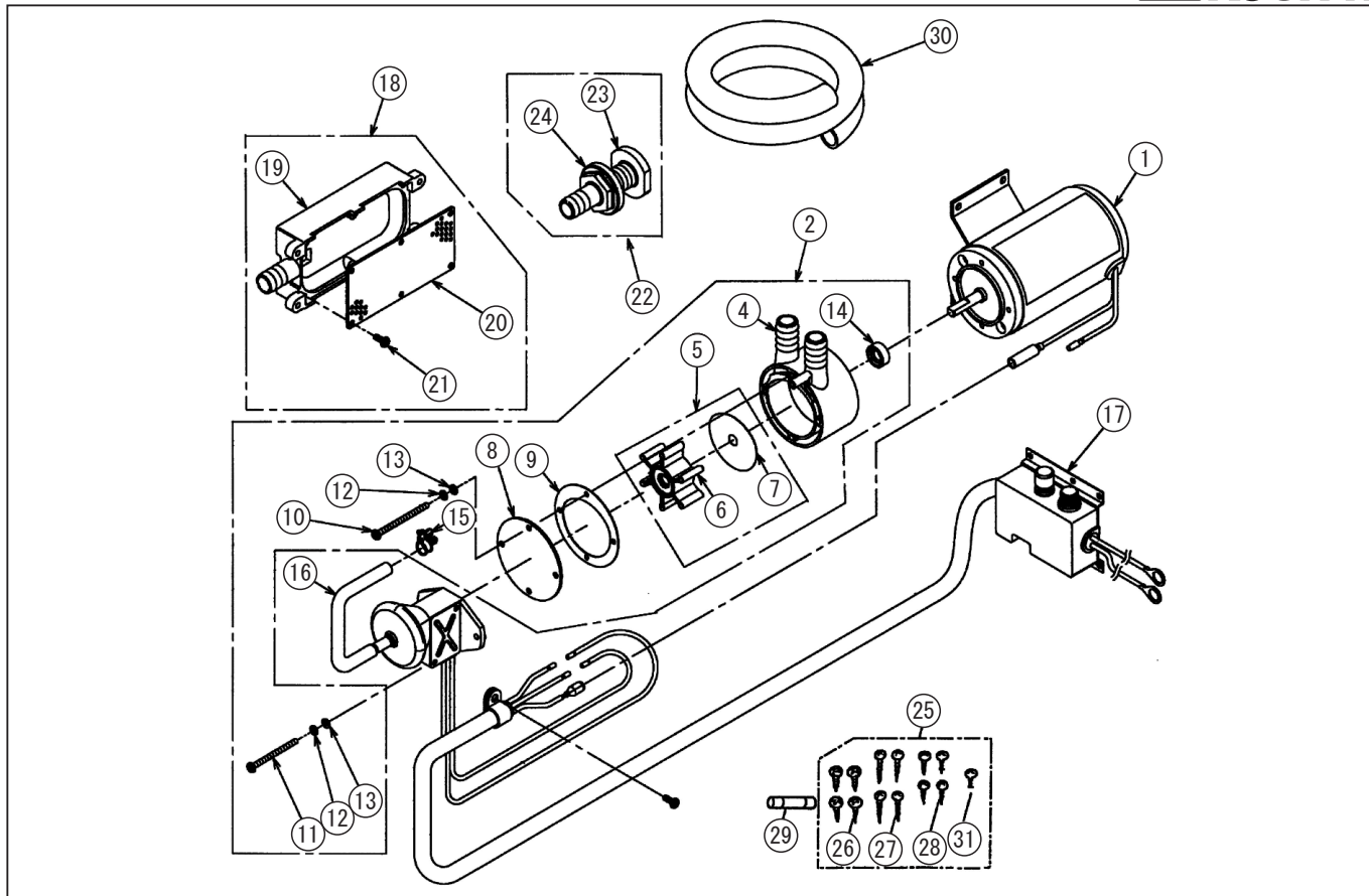
型式名 BK-12/24-2 (029850116/029850216)
