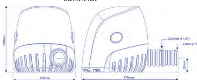
ORCA AUTO 1300
