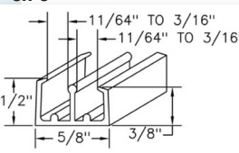
CH-3
